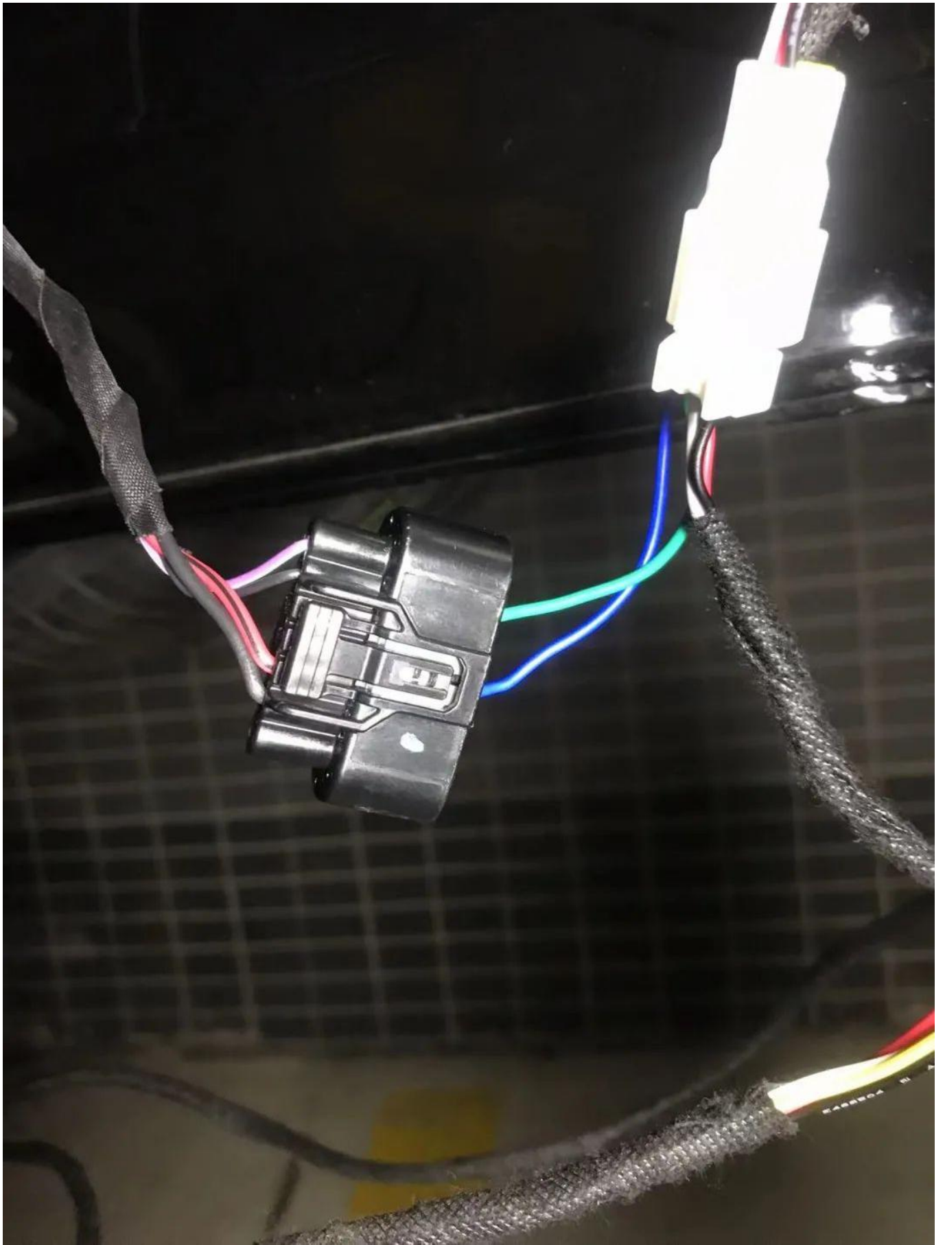
5.尾门开关安装位置
